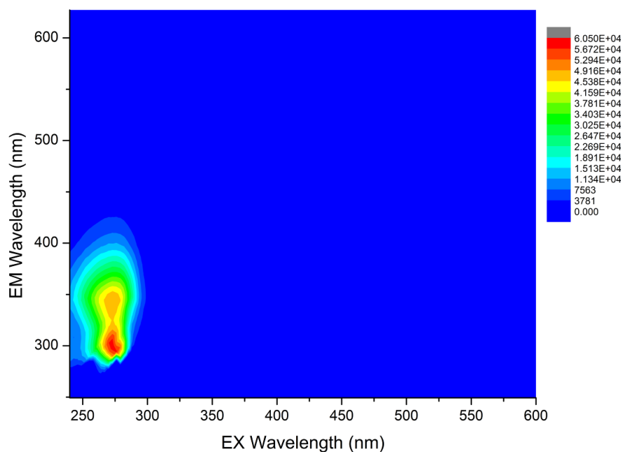
Abbildung 30: EEM von konzentriertem Spurenstoffmix analog zur mittleren Zusammensetzung im IN
