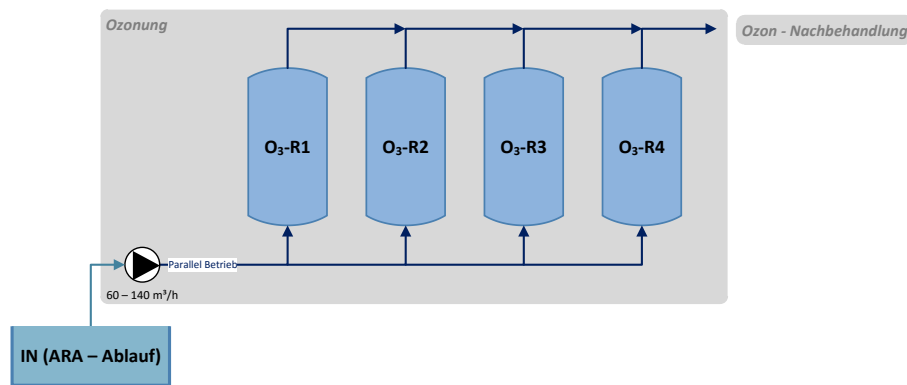
Abbildung 6: Konfiguration der Ozon-Reaktoren im parallelen Betrieb
