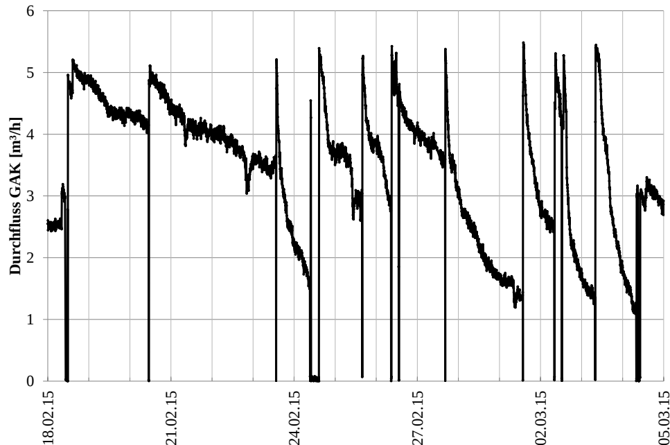
Abbildung 21: Volumenstrom [ \text{m}^3/\text{h} ] zum Aktivkohle-Druckfilter (Stand-Alone) in der Zeit vom 18.02.2015 bis 05.03.2015 ( Q\text{-Soll} = 5 \text{ m}^3/\text{h} )
