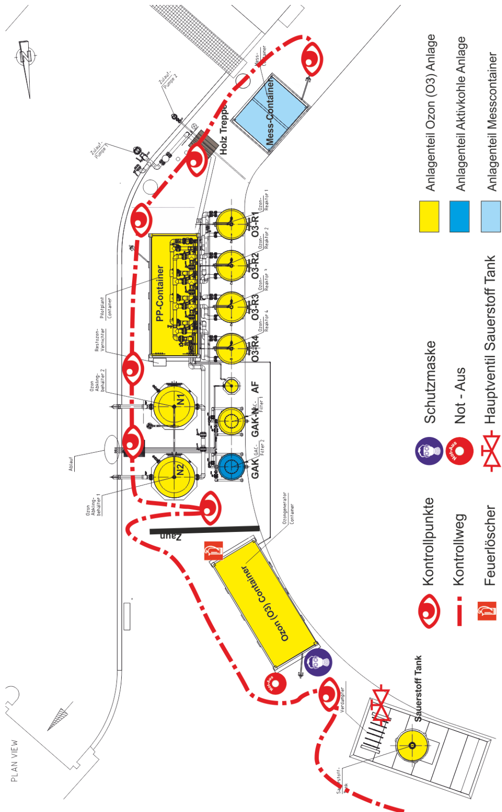
Abbildung 78: Grundriss Versuchsanlage sowie Weg der Routine-Inspektion
