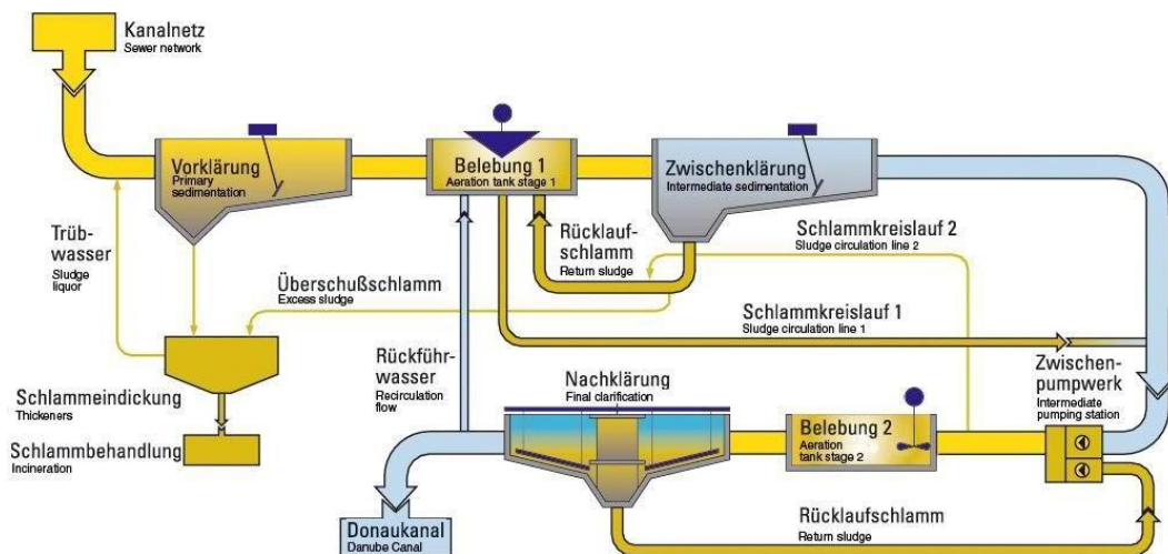
Abbildung 3: Übersicht über das Hybrid ® -Verfahren
