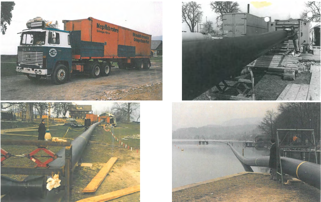
Abbildung 17: Produktion der „Endlosrohre“ in den 1970er-Jahren mit Hilfe mobiler Anlagen und Lagerung der Rohrstränge im See (Bildquelle: RV Attersee).
