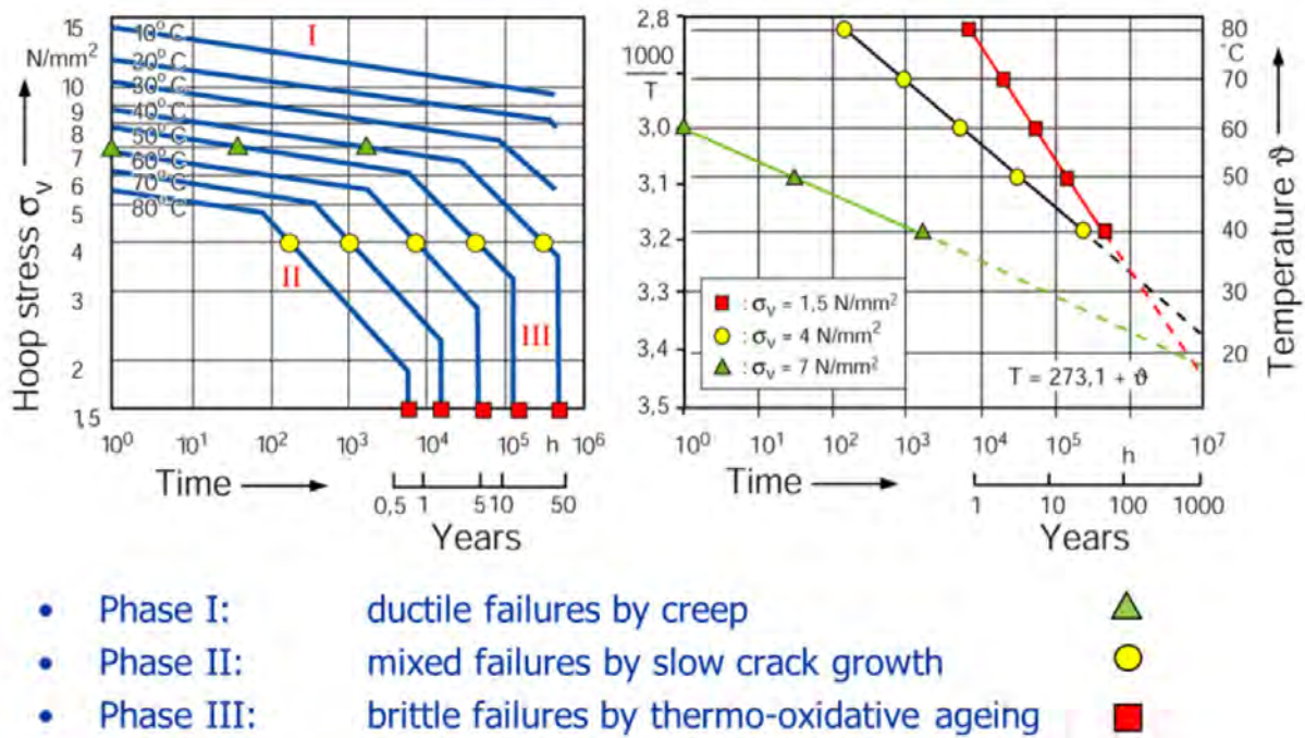
Abbildung 25: Polyethylenrohr: Prinzip eines Zeitstanddiagramms und der Arrhenius-Auswertung (1 MPa = 10 bar = 1 N/mm²) (Meijering et al., 2014).
