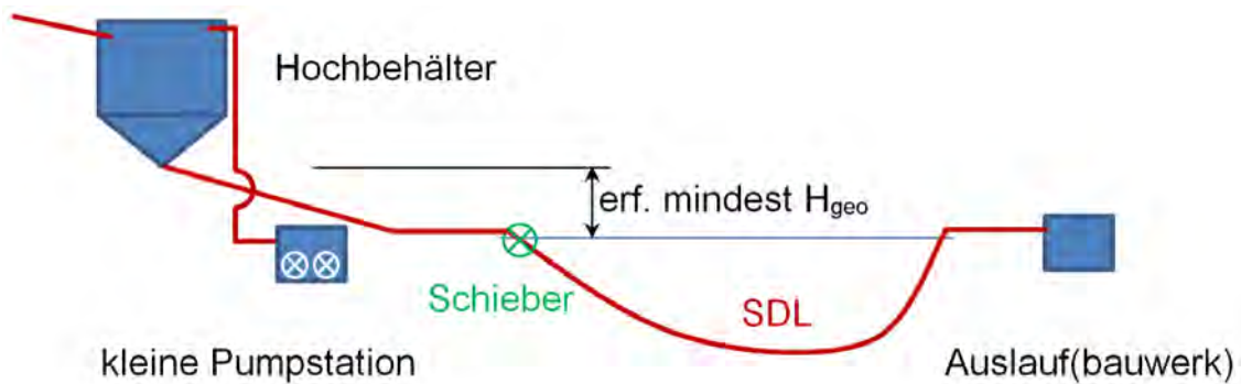
Abbildung 27: Abwassertransport durch die SDL in Freigefälledruckleitungen (optional mit kleiner Pumpstation zum befüllen des Hochbehälters).
