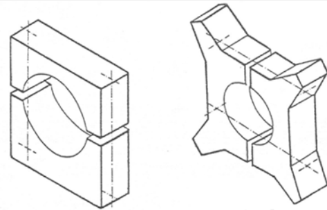
Abbildung 12: Bauformen unterschiedlicher Beschwerungsgewichte für SDL aus PE (Bildquelle: Brömstrup, 2001).
