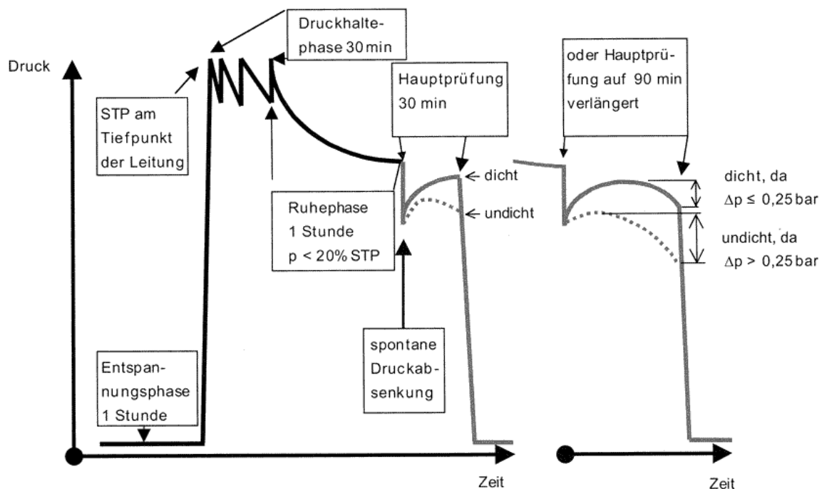
Abbildung 56: Beispiel eines Druckverlaufs beim Kontraktionsverfahren (URL: www.weitbrechtrrohrleitungsbau.de [15.04.2015]).
