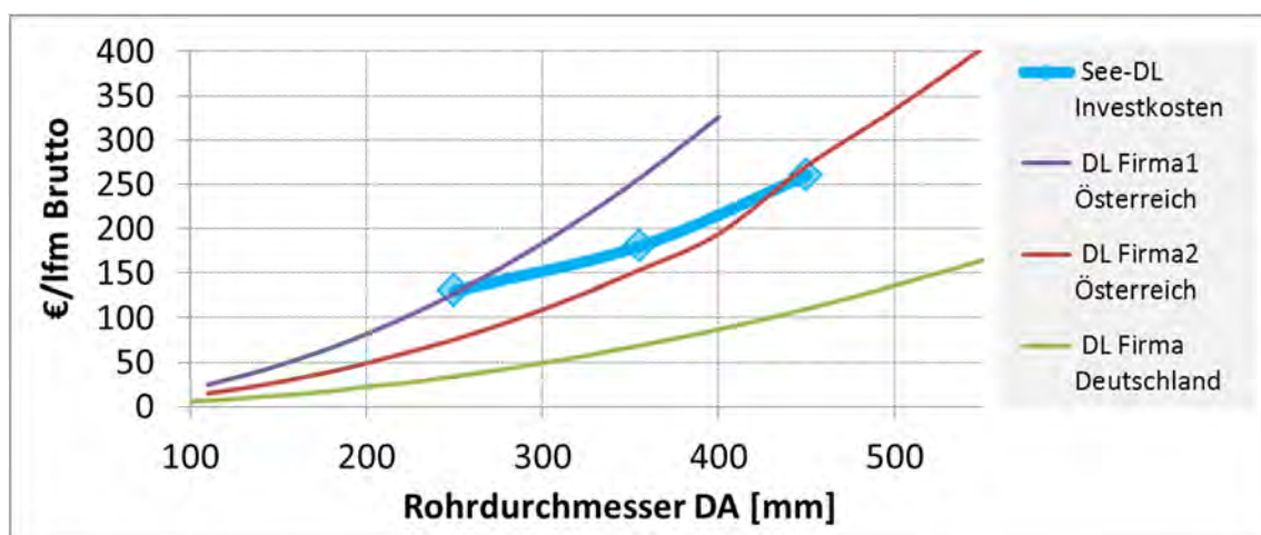
Abbildung 68: Vergleich der indexangepassten Investitionskosten einer Seedruckleitung (See-DL) (Rohrkosten + Kosten der Beschwerungsgewichte) mit Rohrkosten verschiedener Produzenten (DL-Firma) aus den Bruttopreislisten von 2014.
