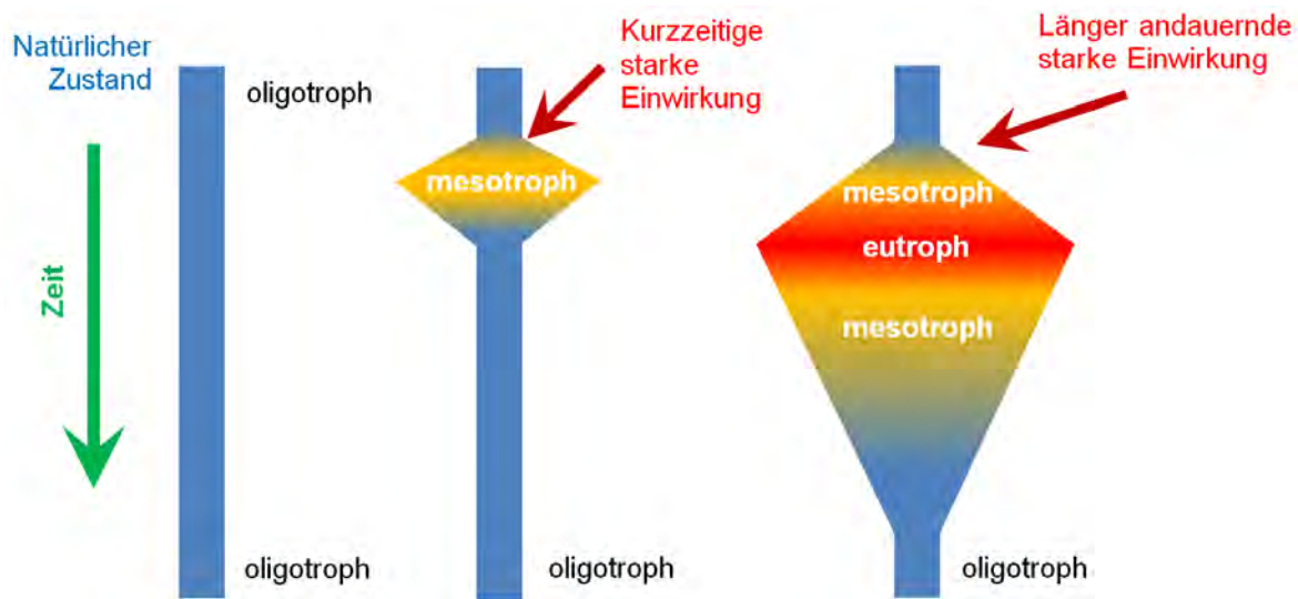
Abbildung 36: Darstellung der Auswirkungen von kurzzeitigen und länger andauernden Einwirkungen (Nährstoffbelastung) auf die Trophie eines Seenwasserkörpers.
