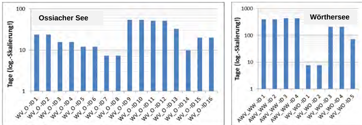
Abbildung 43: Theoretische Anzahl an Tagen pro Seedruckleitung ID_X welche ausreicht, um die Konzentration des Gesamtposphors im See um max. 1,0 µg/L zu erhöhen. (Annahme: Querriss der SDL, Seeinhalt durchmischt). Links: Ossiacher See +0,3 µg/L TP, Rechts: Wörthersee +0,7 µg/L TP.
