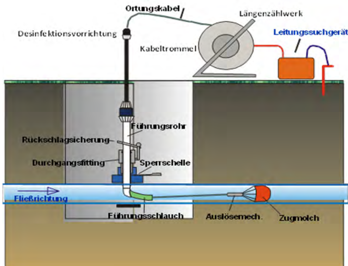
Abbildung 58: Einschwemmverfahren (Unterdechler, 2014).
