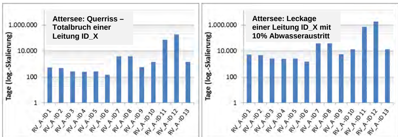
Abbildung 44: Theoretische Anzahl an Tagen pro Seedruckleitung ID_X welche ausreicht, um die Konzentration des Gesamtposphors im See um max. 1,0 µg/L zu erhöhen. (Annahme: Attersee, Seeinhalt durchmischt.). Links: Querriss der SDL; Rechts: Annahme einer Leckage mit Verlust von 10% des täglich gepumpten Abwassers. Hinweis: die Seedruckleitung RV_A ID 14 liegt im Mondsee und wurde bei der Darstellung nicht berücksichtigt.
